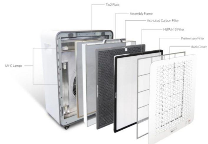
KTIII Air Steriliser
